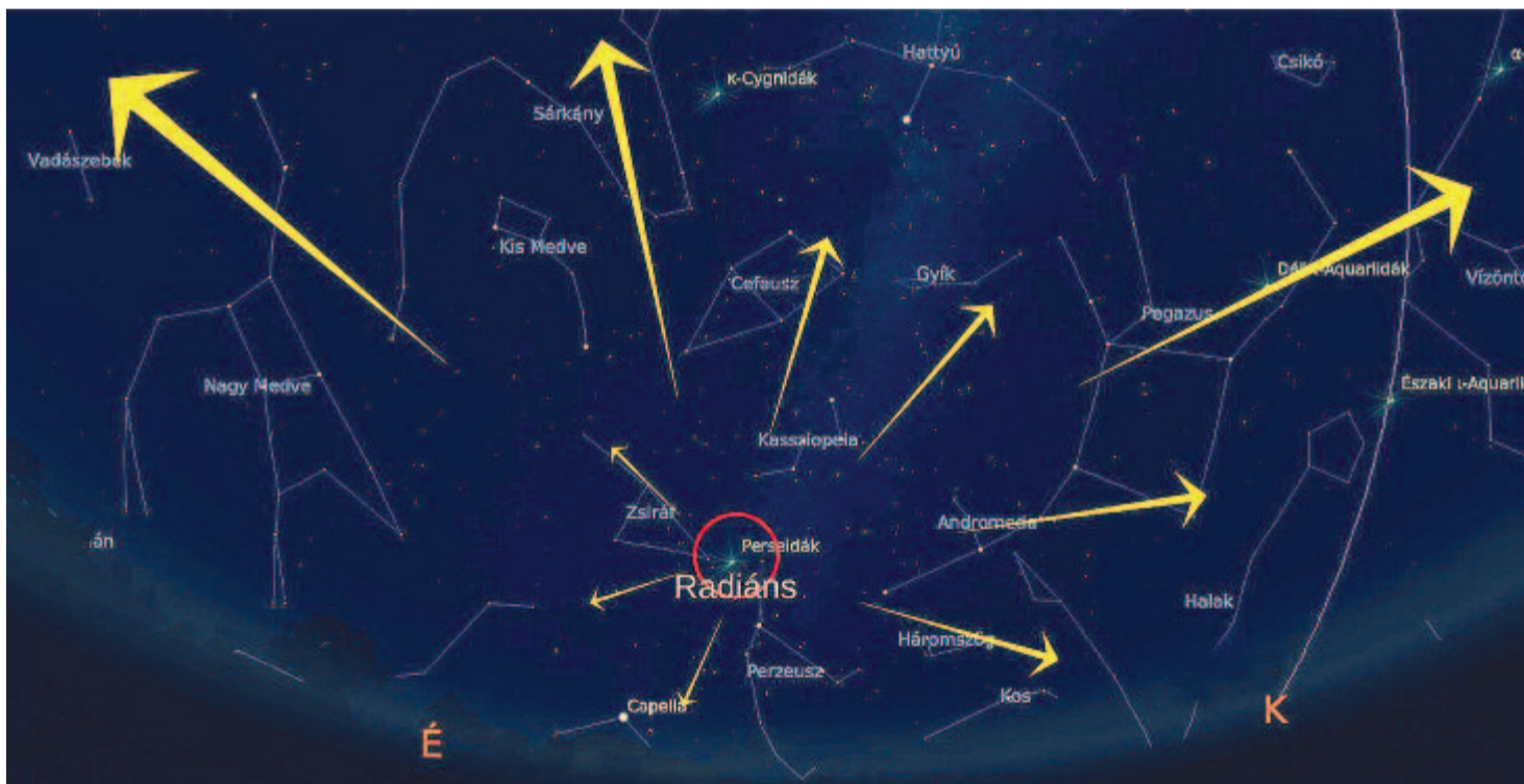
Perseidák
